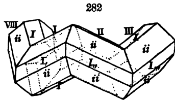
Rutile.
